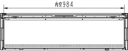
截面 XSEC0002-XSEC0002
