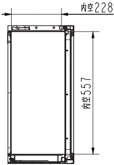
截面 XSEC0001-XSEC0001
